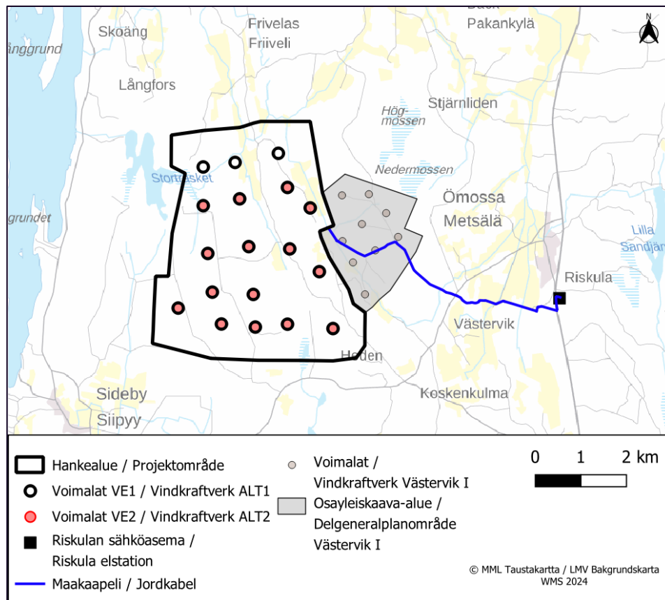
Bild 1. Alternativen ALT1 och ALT2 samt projektets elöverföring som bedöms i förfarandet vid miljökonsekvensbedömning.
