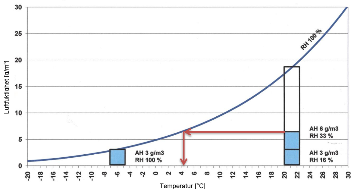
Bild 1. Mättningskurva (RH 100 %) för luftens relativa fuktighet som en funktion av luftens temperatur. (Källa: Karnaattu & Pesonen)
